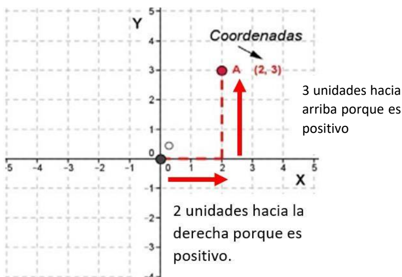
Imagen N° 5. Coordenadas. Fuente: Imagen de Elaboración Propia
