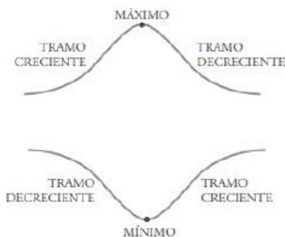
Imagen N° 19. Máximos y mínimos. Fuente: Imagen desconocida
