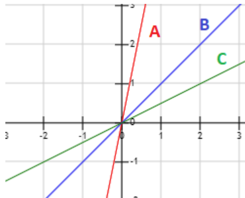
Imagen 33: Funciones lineales.
