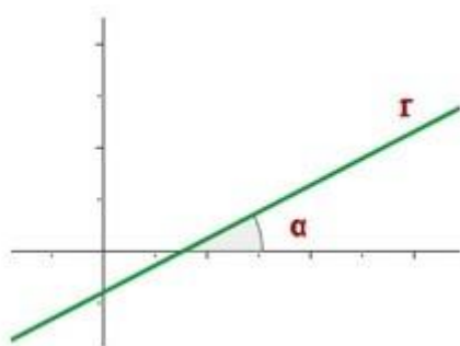
Función CRECIENTE m > 0
