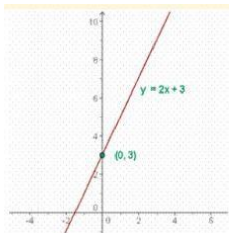
Imagen 35: Función lineal
