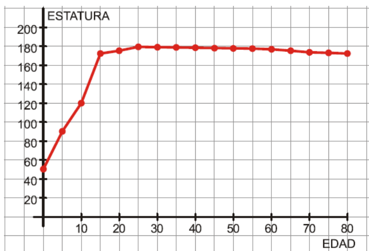
Imagen 27: Gráfica.
