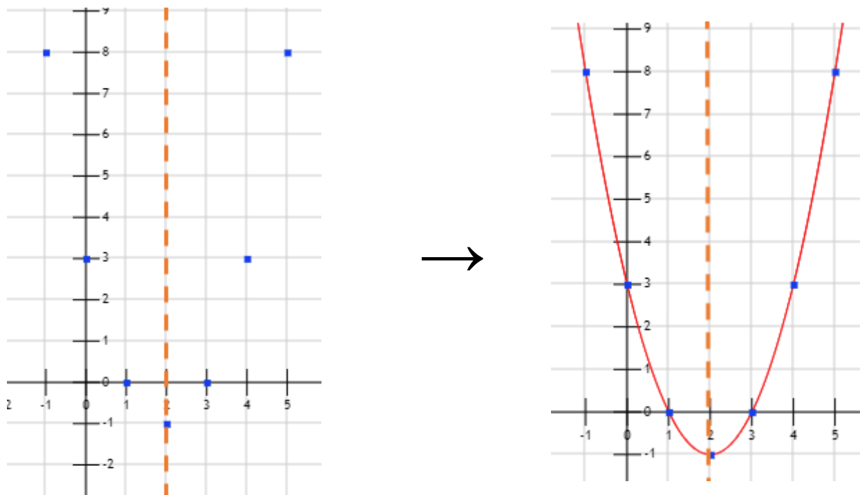
Imagen 45: Representación de una función cuadrática.
