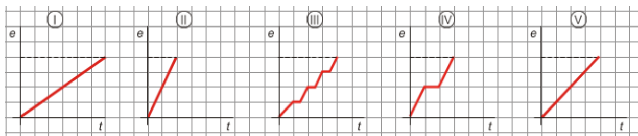
Imagen 26: Gráficas.
