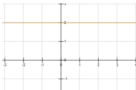
Imagen 38: Gráfica función constante.
