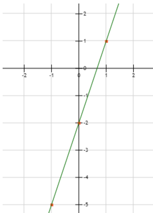
Imagen Nº 10. Gráfica. Fuente: Imagen de Elaboración Propia
