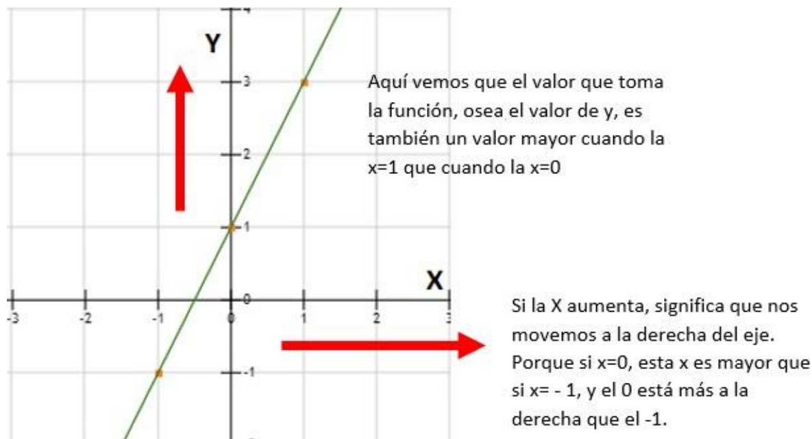
Imagen N° 15. Gráfica Creciente. Fuente: Imagen de Elaboración Propia
